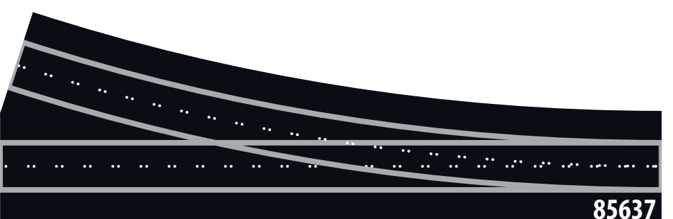
85637 : Aiguillage à droite en voie étroite, 128 mm de long, rayon de 409 mm, 18° de déviation
